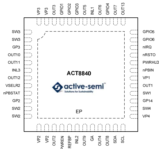
Thin - QFN (TQFN66-48)
